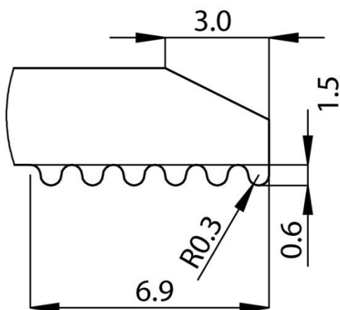
Einzelheit A Maßstab 4:1
