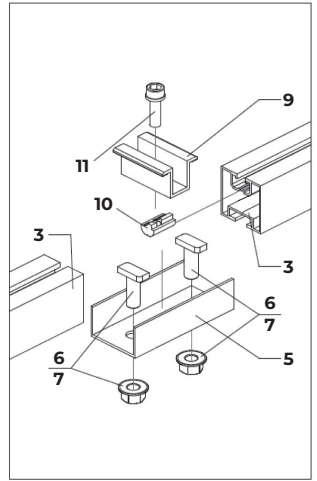
Einzelheiten C
