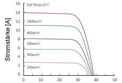
Spannung [V] Modulleigenschaften bei konstanter Modultemperatur von 25°C und variabler Bestrahlungsstärke
